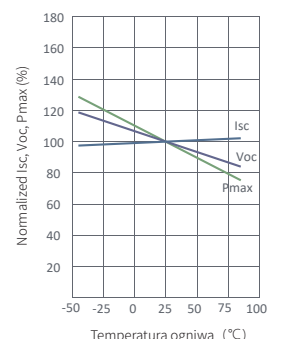
Charakterystyka zmiany mocy w funkcji temperatury ogniw
