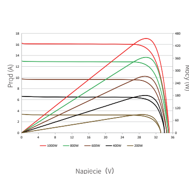
Charakterystyka prądowo – napięciowa (445W)
